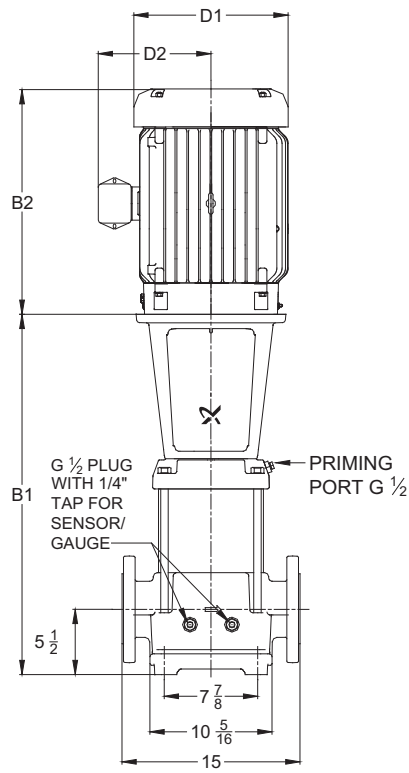
4-5 STAGES 4" ANSI 250 LB R.F.
