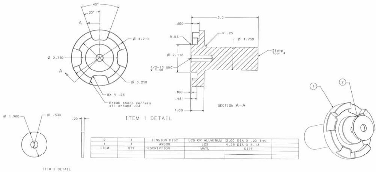
CFR / ETFE Impeller Trim Arbor (PT0827) Fig. 11-9
